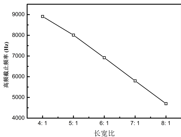
Figure 2: 声场旋转器高频截止频率与长方体结构单元长宽比的关系
