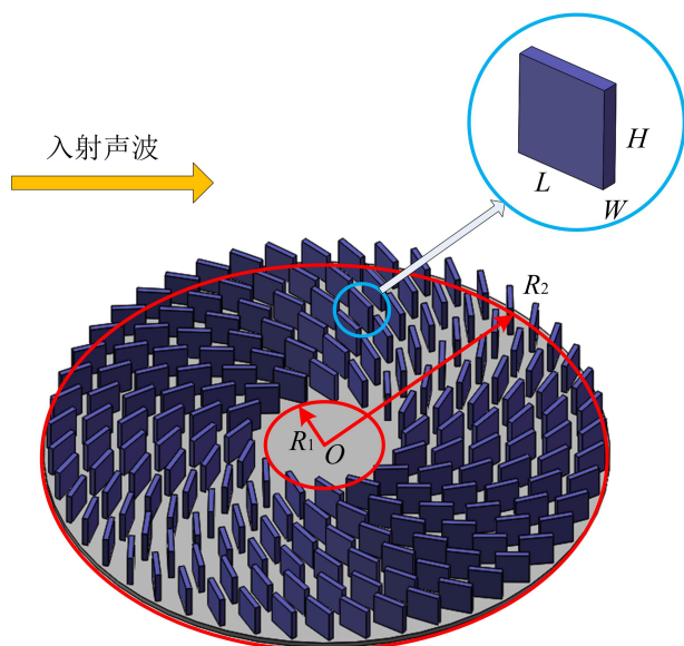
Figure 1: 声场旋转器结构示意图
